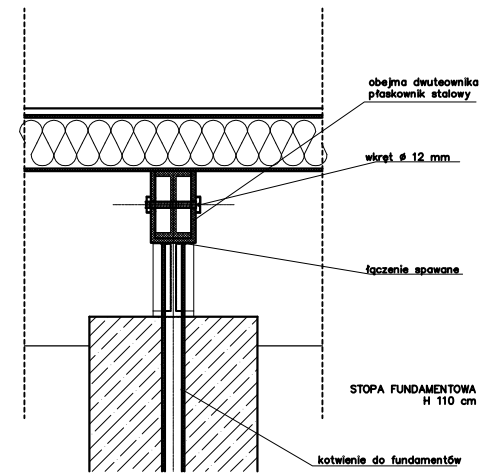
DETAL KOTWIENIA DWUTEOWNIKÓW
